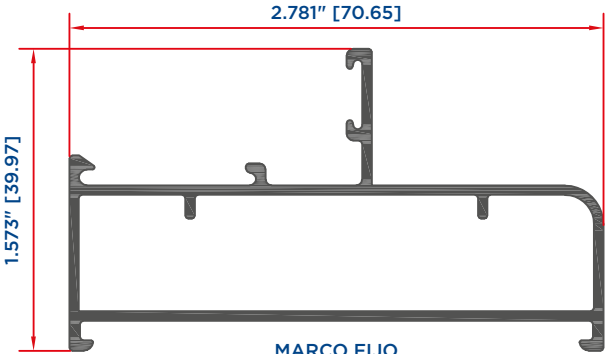
MARCO FIJO 1618
