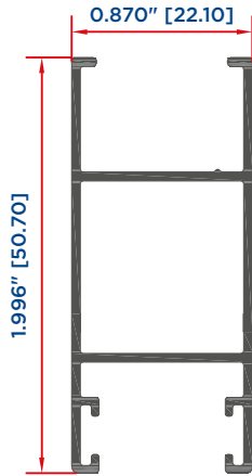
CERCO DUO 12157
