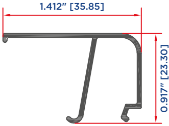
JUNQUILLO REDONDO 12012
