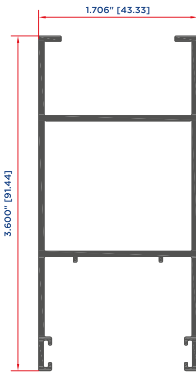
CERCO DUO 12311
