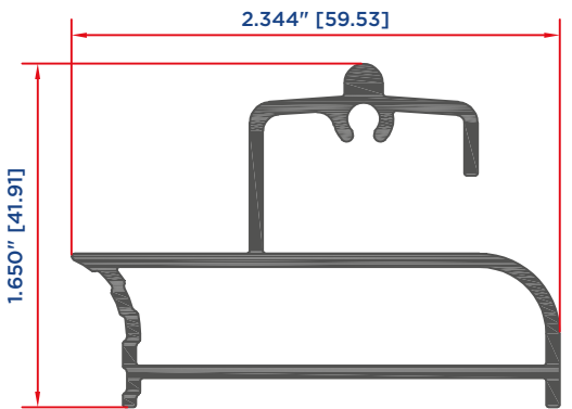
ADAPTADOR RIEL 12304
