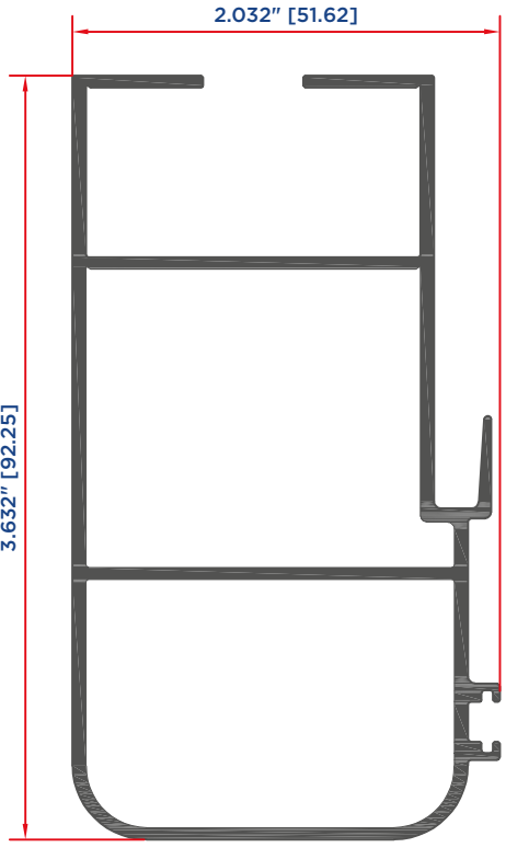
TRASLAPE 12309
