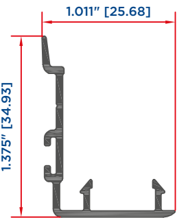
ADAPTADOR TRASLAPE 1619
