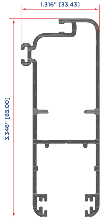
MOSQUITERO PUERTA 2198
