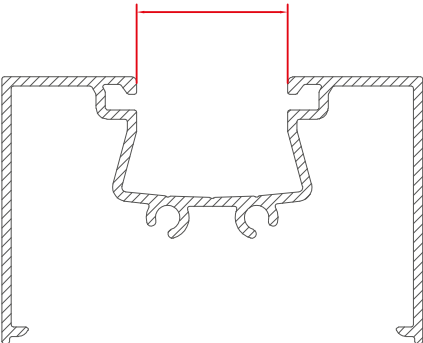
BOLSA DUO 2304
