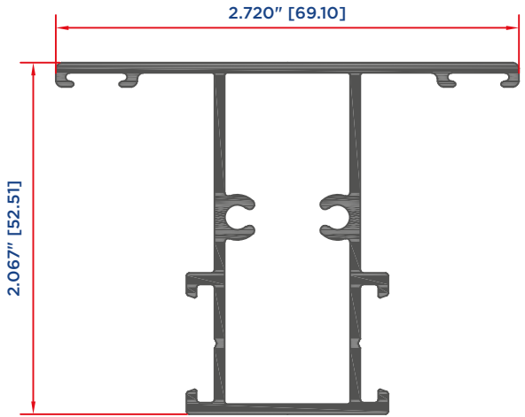
INTERMEDIO 12015
