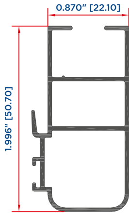
TRASLAPE 12155
