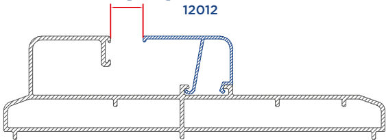
FIJO 12014
