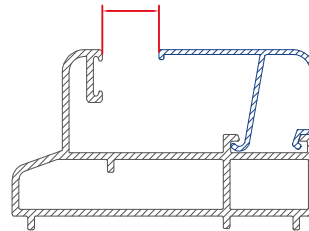
FIJO 12009
