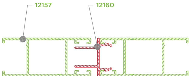
Ensamble del perfil OXXO 12160.
