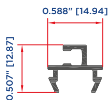
ADAPTADOR MOSQUITERO 12315
