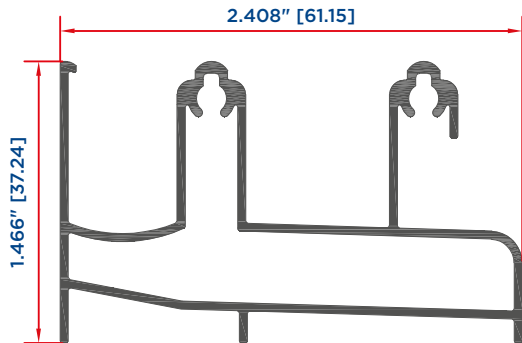
RIEL INFERIOR 12150
