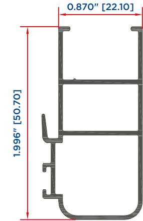
TRASLAPE DUO 12158
