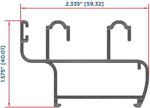
RIEL DOBLE 1695
